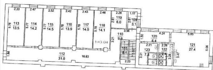
План этажа 1
