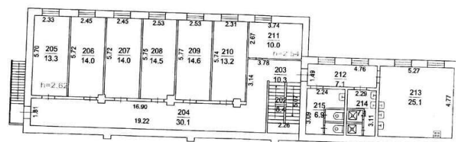
План этажа 2
