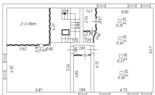
План 3 этаж
