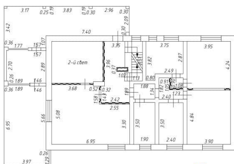
План 2 этаж
