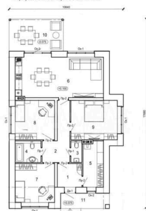
Маркировочный план первого этажа М 1:100
