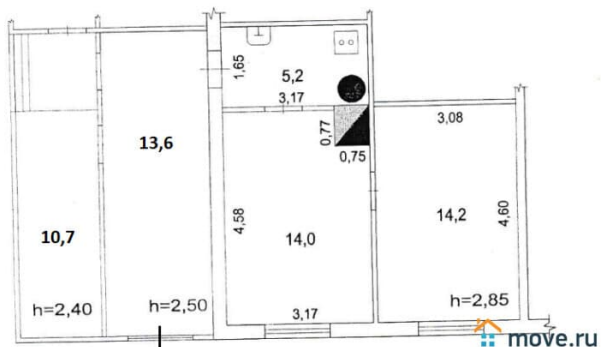
План дома (фактическая площадь)
