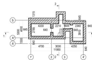
Подвал
