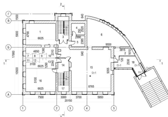
1 этаж
