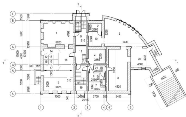
Цоколь
