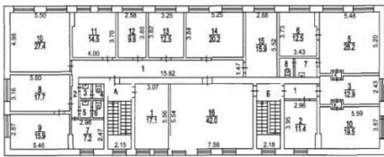
ЭТАЖ 2 - 349,6 м² (по БТИ)
