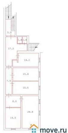
2 этаж
