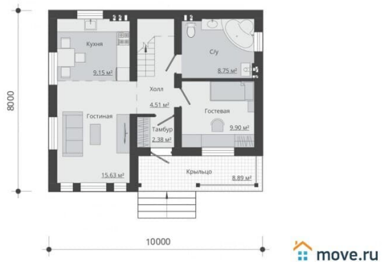
План 1 этажа
