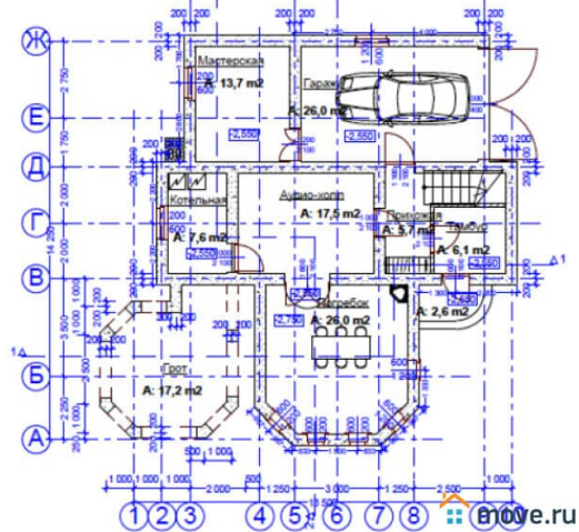
План цокольного этажа на отметке -2.550
