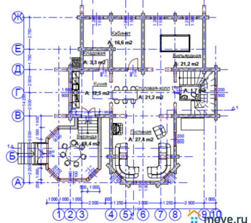
План 1 этажа на отметке 0.000
