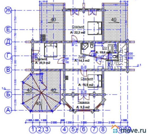
План 2 этажа на отметке +3.150
