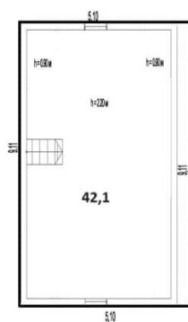
План 2 этаж
